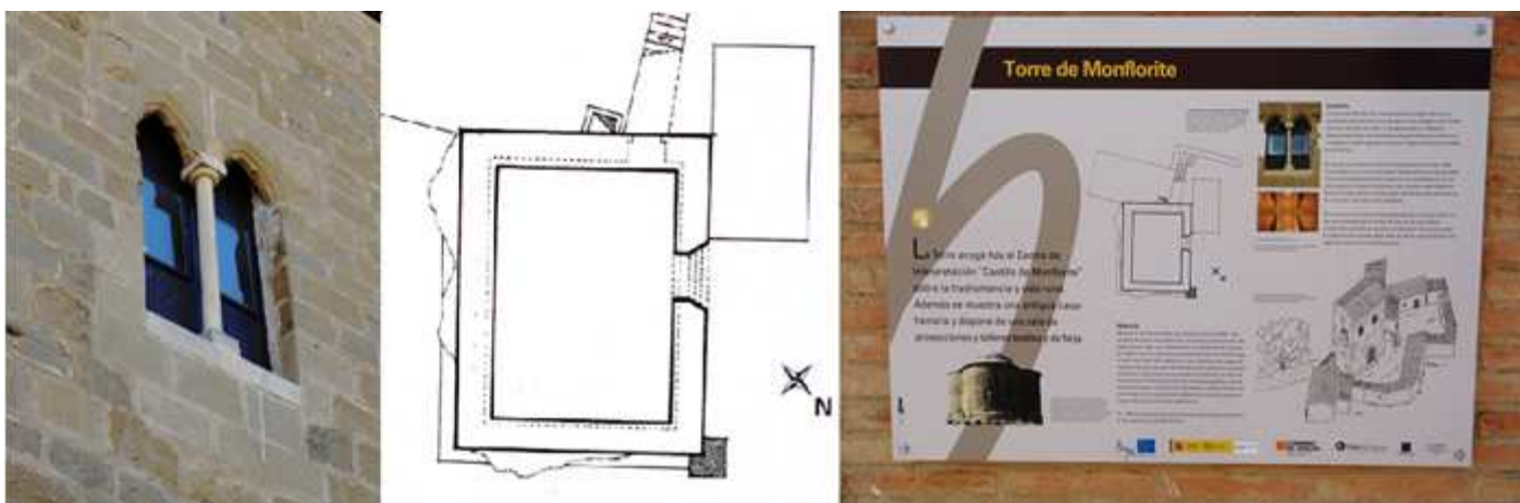
❶ Detalle de las ventanas de la fachada principal. ❷ Croquis de la torre del cartel informativo. Con una planta de 10 por 8m. ❸ Cartel informativo con una recreación del conjunto de la torre y las edificaciones en la edad media.
